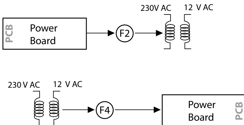
Fig. 16 Wiring diagram
