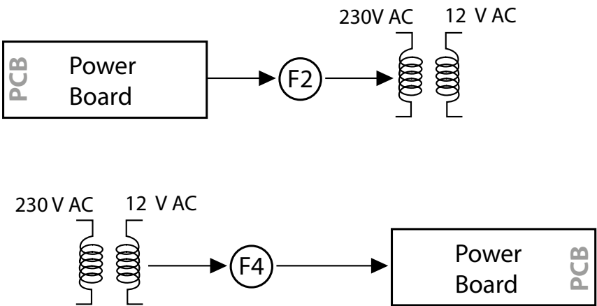
Fig. 14 Wiring diagram
