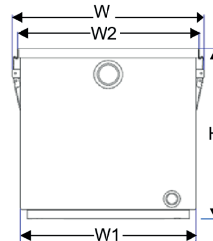
VISTA LATERAL
